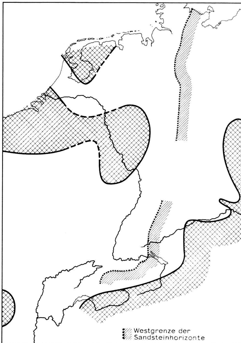
Fig. 7. Vermutliche Verteilung von Land und Meer im Unteren Lias und Westgrenze der Verbreitung von kompakten Sandsteinhorizonten vor der Ostküste.
