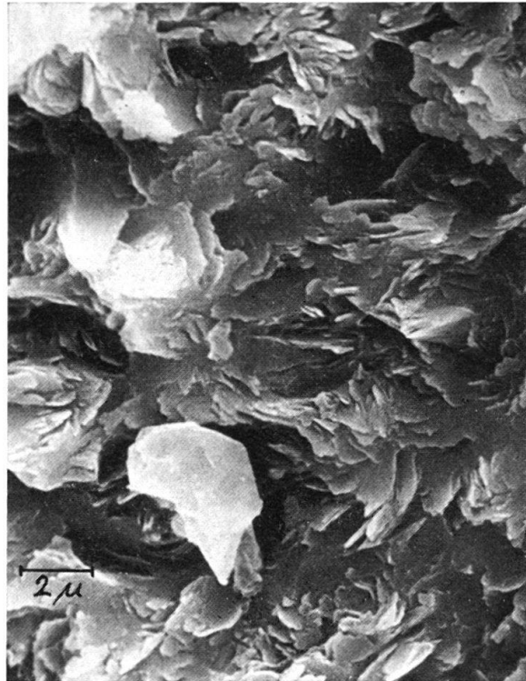
Fig. 20. Gebrochenes, angeätztes Glaukonitkorn. Stereoscan-EM, Probe P/16.
