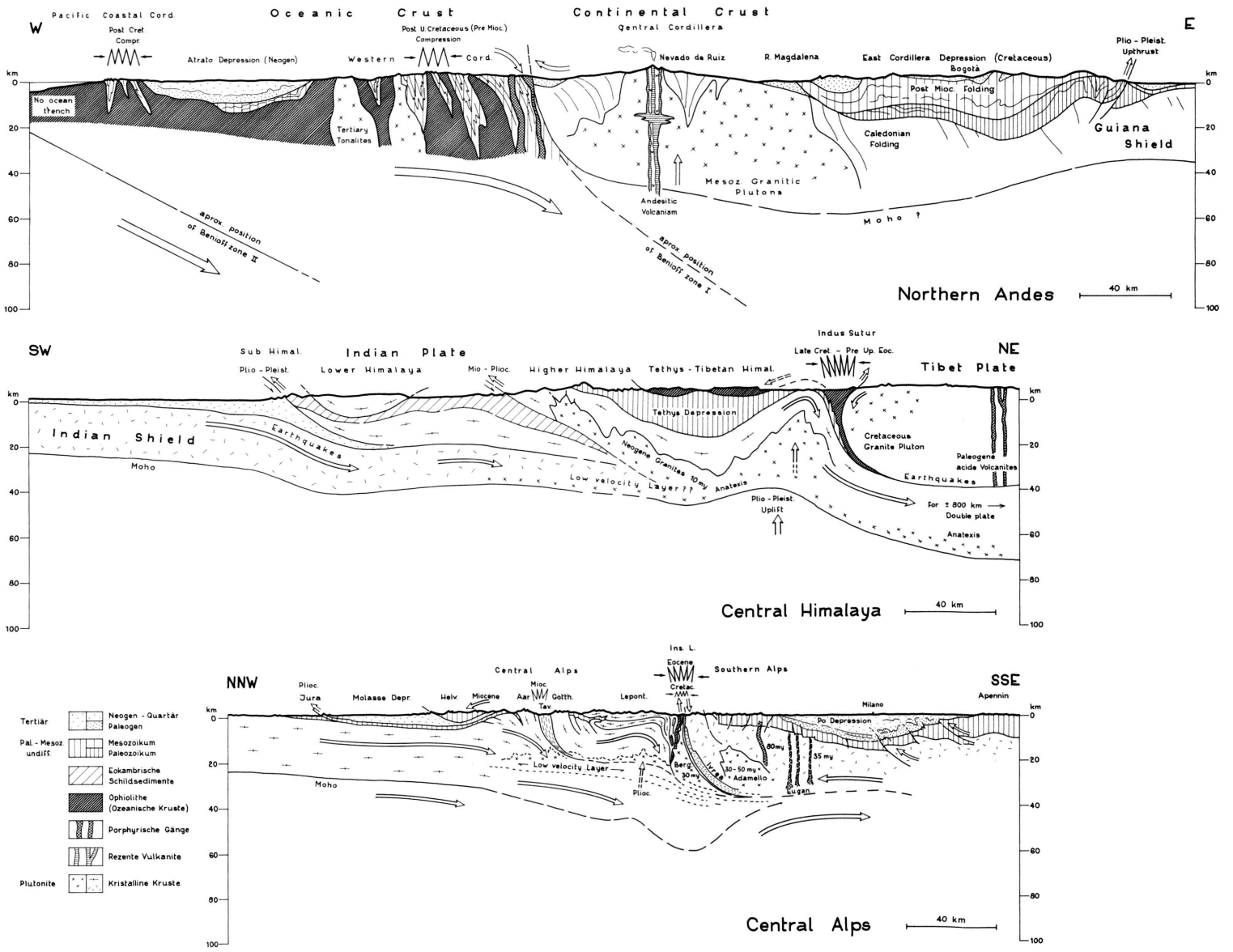
Strukturprofile durch die Anden, Himalaya und Alpen
