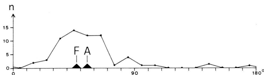
Fig. 7. Directions des fissures à remplissages colorés de St-Triphon. n: nombre de fissures par intervalle de 10° (65 mesures; carrière du Lessus). A: failles conjuguées des Andonces. F: grande faille des Fontenailles.
