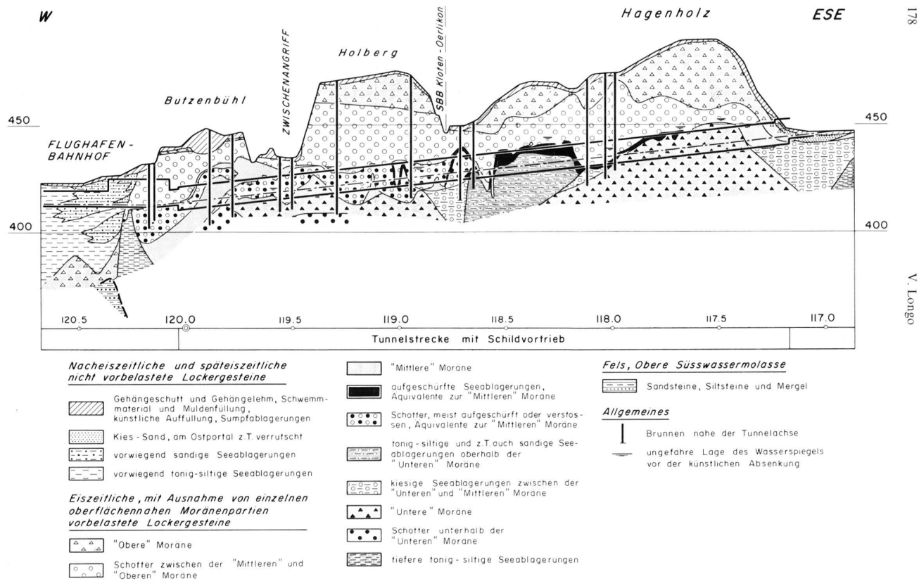
Fig. 2. Geologisches Längsprofil des Hagenholztunnels (10× überhöht).
