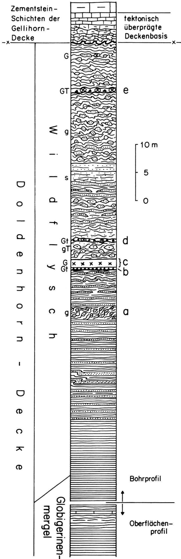
Fig. 3. Profil der Kernbohrung Gamchi (Kiental) durch die Basis der Gellihorn-Decke und den Flysch der Doldenhorn-Decke.
