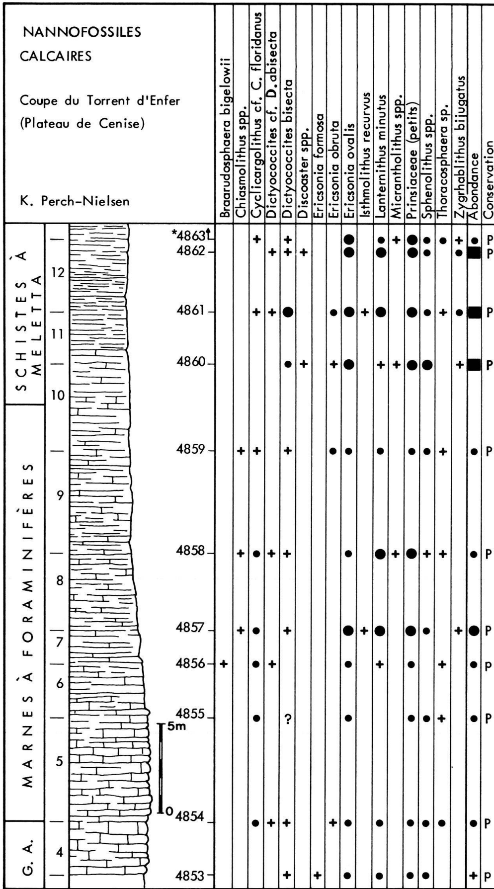
Fig. 16. Distribution des nanfossiles calcaires dans la coupe du Torrent d'Enfer (synclinal de Cenise). G.A. = Calcaires gréseux à Grands Foraminifères arénacés.
