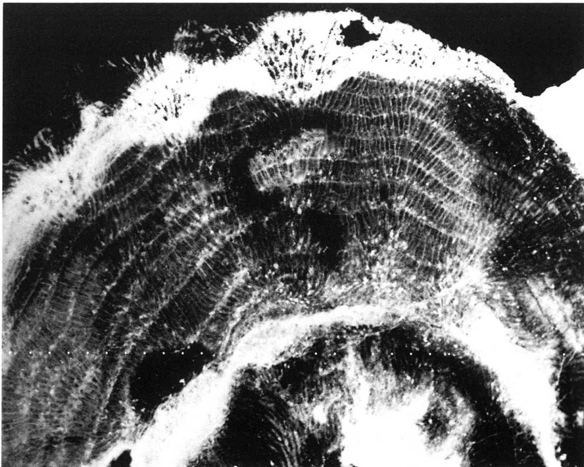
Fig. 9. Ptychochaetetes (Granatiparietes) helveticus n. sp. Vertikalschnitt durch das Coenosteum eines Paratyps. Man beachte die langen Röhrenchen und die deutlichen Latilaminae. A 1021/a. \times 8 .
