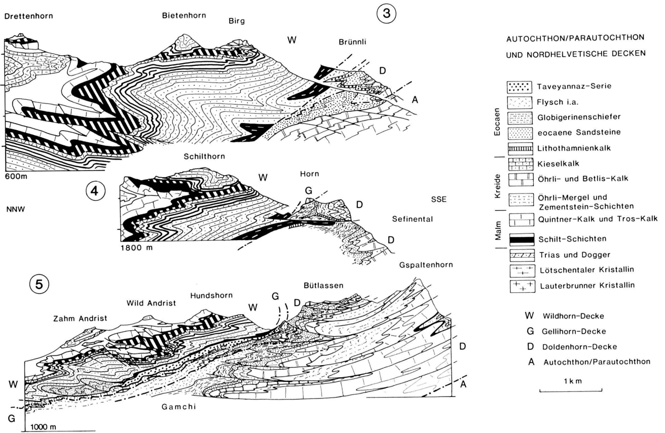
Fig. 1. Profile durch den Nordrand des Aarmassivs und die anschließenden helvetischen Decken zwischen Eiger und Kiental.
