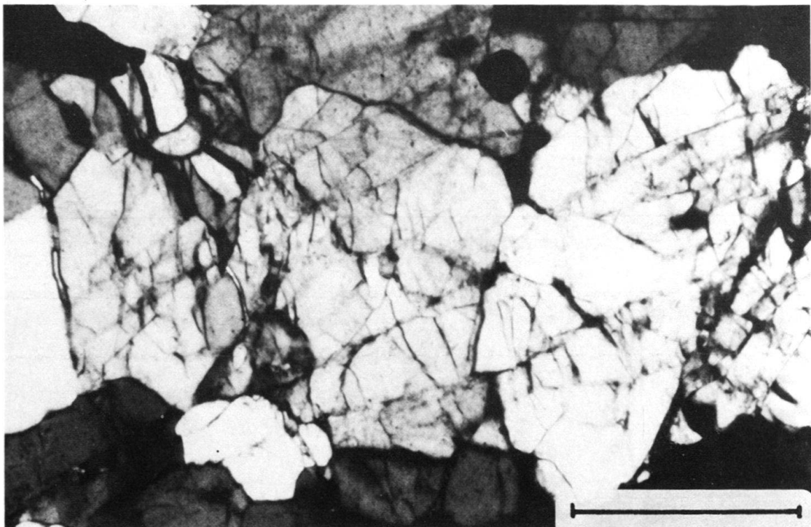
Fig. 3. Katakklase im Cacciola-Granit: Normaltypus – Granit mit starker Katakklase in den Quarzkörnern. Furkattunnel (UR), 3563 m ab Ostportal. Photo Nathist. Mus. Bern, P. Vollenweider. Maßstab = 0,5 mm.
