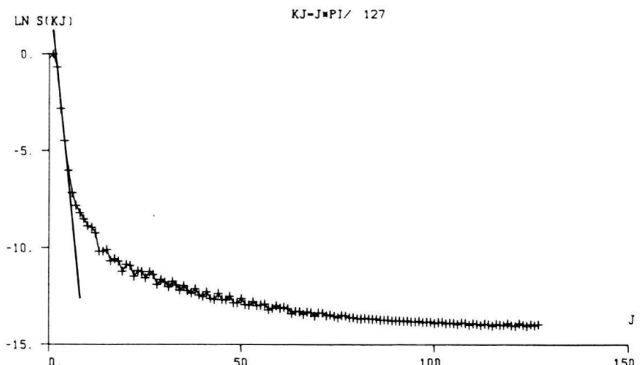
Fig. 1. Exemple de spectres de puissance, S(kj) , en coordonnées semi-logarithmiques, obtenus par FFT sur les anomalies résiduelles du champ magnétique (Champ total). Les graphiques comportent les droites, de pente H = 2h/\Delta x , tracées lors de l'interprétation et ayant servi à la détermination des profondeurs.
