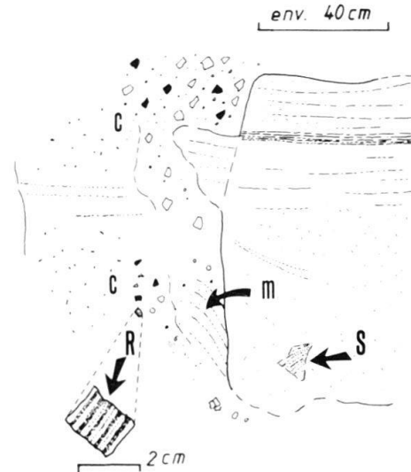
Fig. 12. Cornieule dolomitique polymictique et structures karstiques.
