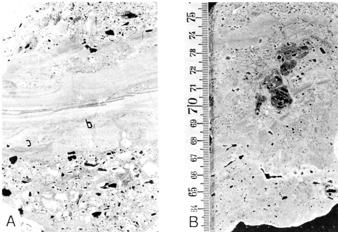
Fig. 11. Association intime de la cornieule dolomitique monomictite, des structures karstiques et des remaniements progressifs et continus.
