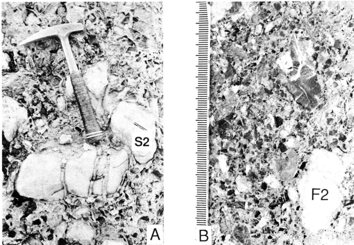
Fig. 6. A. Cornieule dolomitique monomictite d'aspect cloisonné. Les cloisons de sparite qui recourent la schistosité principale (soulignée par S2) des dolomies, prouvent leur postériorité par rapport aux mouvements alpins. Pennique à Zermatt (VS).
