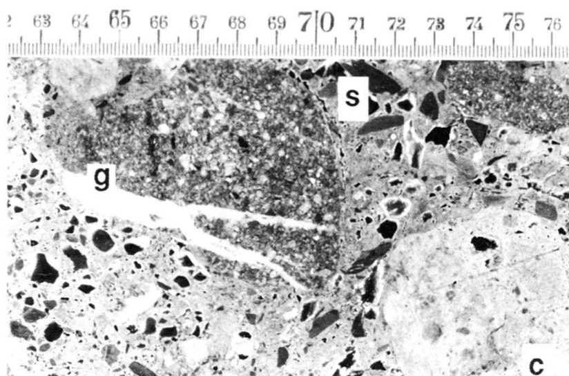
Fig. 7. Section sciée de cornieule dolomitique polymictique à éléments post-triasiques très divers, par exemple: g = Grès de Taveyanne, s = Schistes à Globigérines, c = boules de cornieule dolomitique reconstituées (2 phases). Ultrahelvétique supérieur (nappe de Bex) au col de la Croix (VD).
