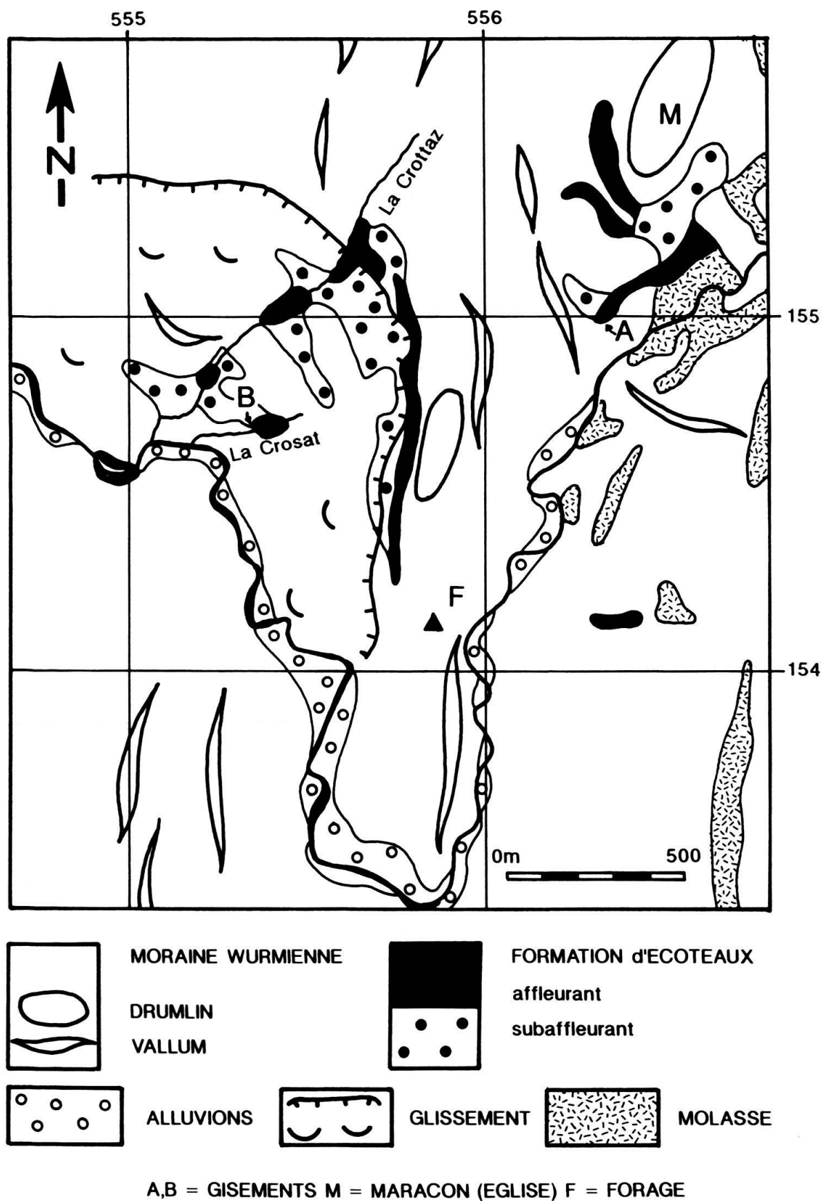
Fig. 2: Carte géologique et morphologique simplifiée du bassin d'Ecoteaux.
