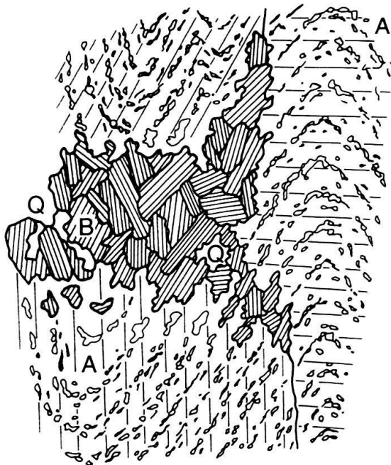
Fig. 5. Postkinematisches Wachstum von Andalusit (A) und Biotit (B) in Metapeliten vom Lägħ da Cavloc. Eine Krenulation wird abgebildet durch Einschlüsse von Biotit, Quarz (Q) und Eisenoxid (Zeichnung modifiziert nach Cornelius 1925).
