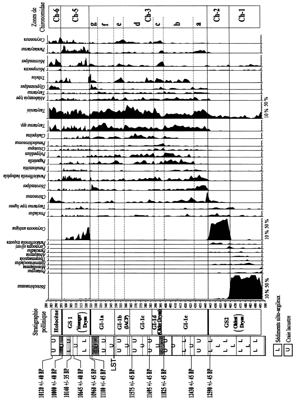
Fig. 2. Diagramme des assemblages de Chironomidae (Lautrety, sondage L6).
