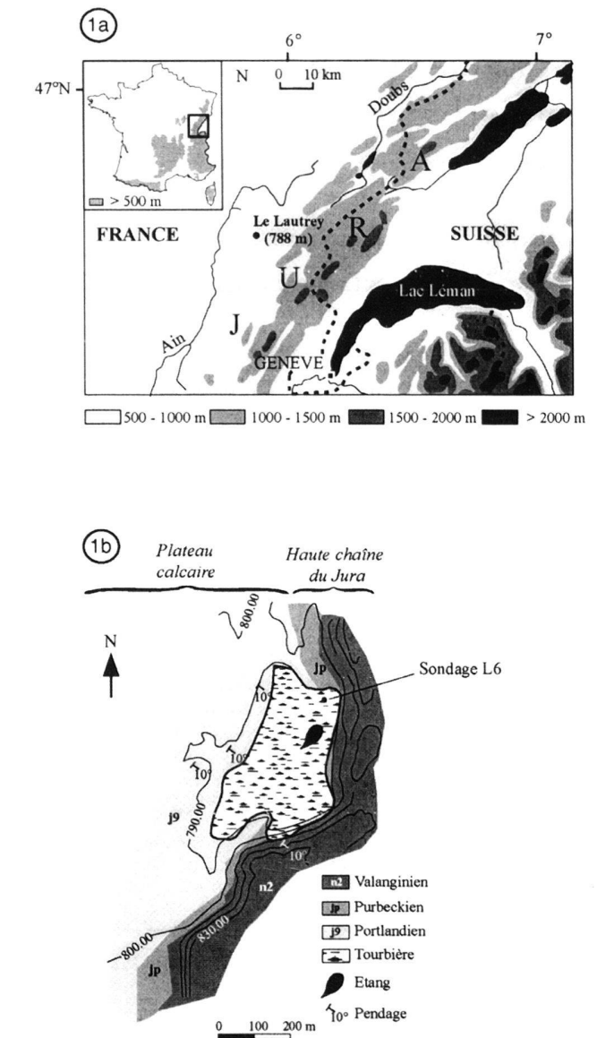
Fig. 1.a. Carte de localisation du site d'étude : le Lac du Lautrey (Jura, France).
