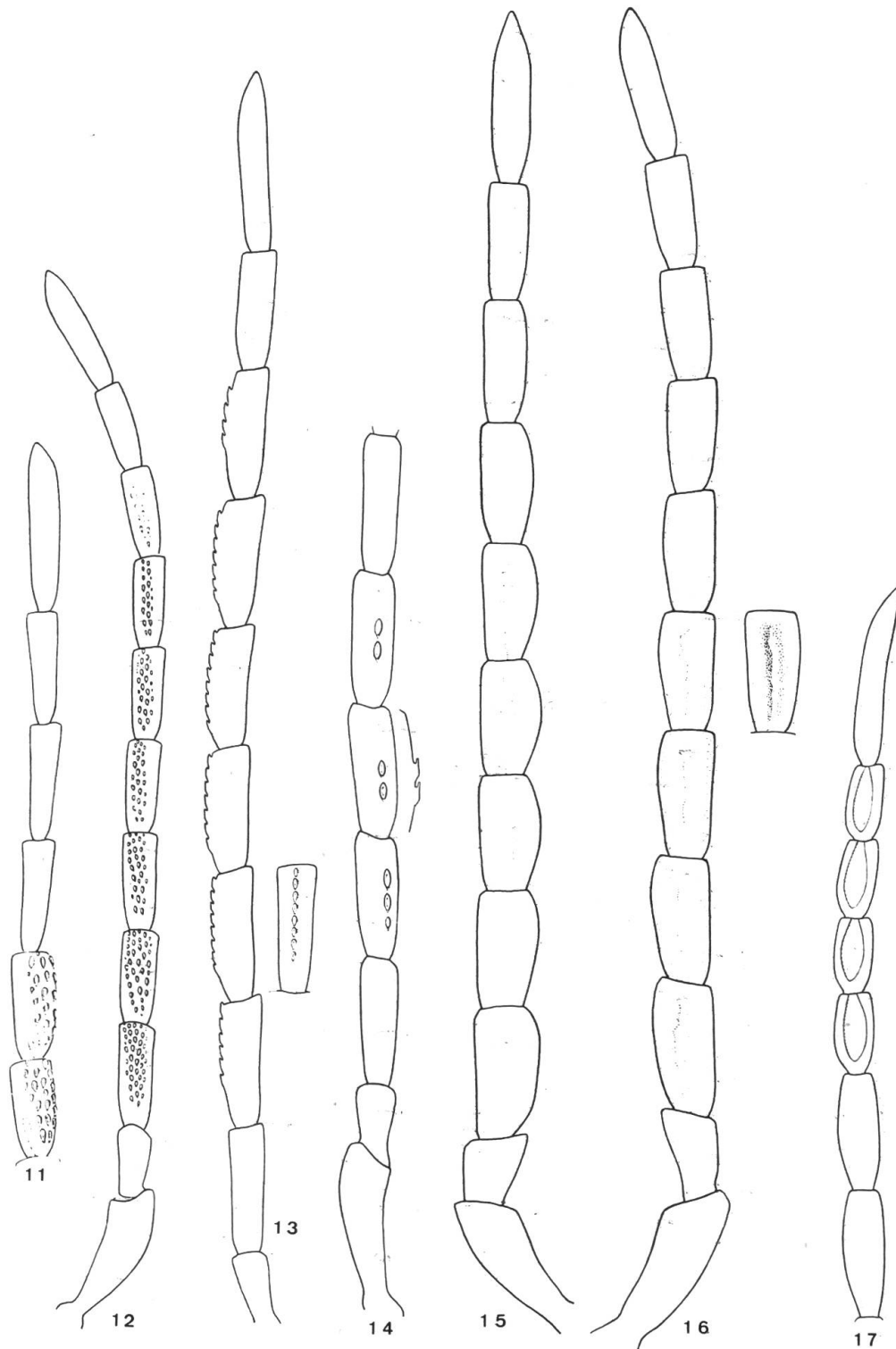
Abb. 11–17: Fühler von Asiosilis ♂: 11, multituberculata n.sp., Glieder 6–11. 12, waterstradti (Pic). 13, tuberculata n.sp., Glieder 2–11, rechts daneben Glied 5 von oben. 14, sparsetuberculata n.sp., Glieder 1–7, rechts daneben Glied 5 im Profil. 15, incarinata (Pic). 16, idem, rechts daneben Glied 6 die Variabilität des Eindrucks zeigend. 17, borneensis (Pic), Glieder 5–11.
