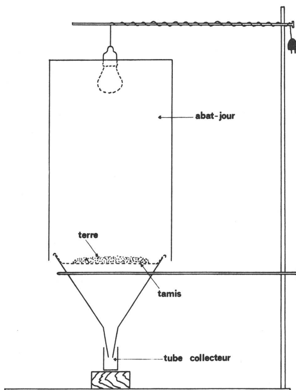
Figure 2 : Modèles de pièges utilisés 2 A: piège lumineux (modèle Changins) 2 B: extracteur de pédofaune
