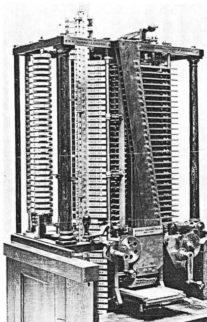
Analytische Maschine mit Ausgabedruker und Lochkarte zur Steuerung
