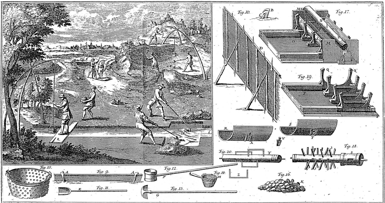
Erzaufbereitung. Aus: Abhandlung von den Eisenhammern und hohen Ofen. Von - von Courtivron und - Bouchu. In: Schauplatz der Künste und Handwerke Bd. 2. Berlin, Stettin, Leipzig, 1763.
