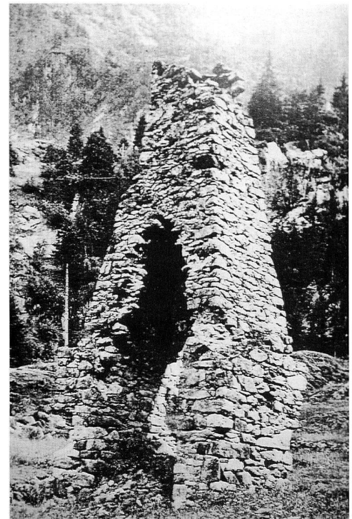
Bild 14: Esse des Trachsellaener Verhüttungssofens vor der Zerstörung durch die Stägen-Lawine 1931. Unterhalb des Sockels, von dem an sich die Esse nach oben verjüngt, befand sich die Flugstaubkammer.
