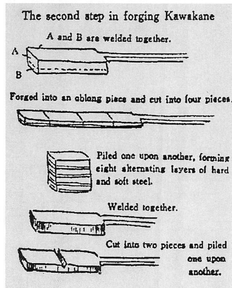
Schema der japanischen Damaszier-Techniken (nach Chikashige, o.c.)
