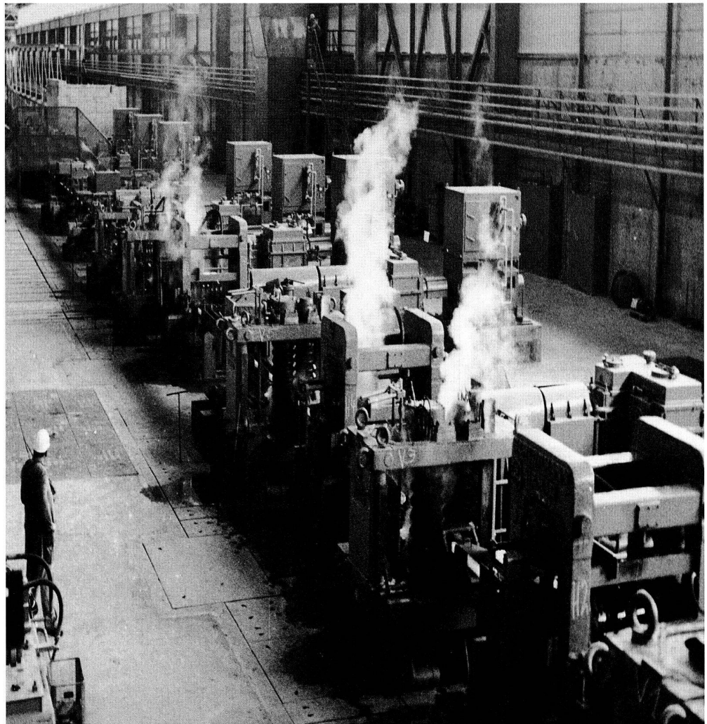
Kombinierte Stab- und Walzdraht-Strasse, 1980. Während der Stahlkrise 1975–1988 nahm das dreiarmlige Warmwalzwerk auf dem Littauerboden (Littau) seinen Betrieb auf. Mit 123 Mio. Franken stellte es die grösste Investition in der von Moos-Geschichte dar.
