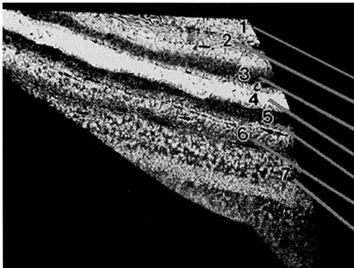
Abb. 19: Streifiges Gefüge in dem Span, welcher der breiteren Schwertklinge unterhalb eines Korrosionsloches entnommen wurde, sowie zugeordnete Mikrohärteergebnisse.
