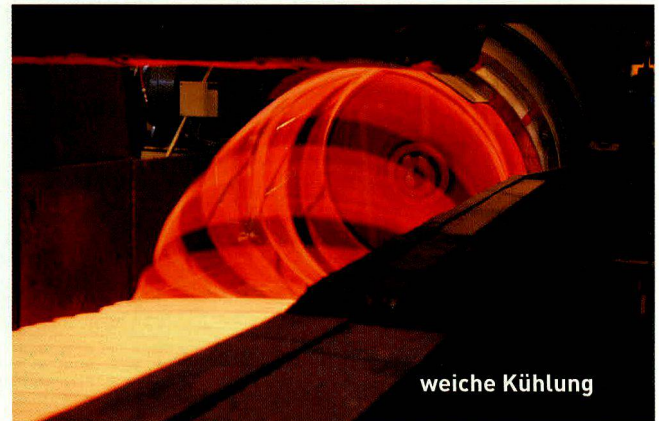
Windungsleger zum Ausfächern des Drahtes auf dem Stelmore-Rollenband.
