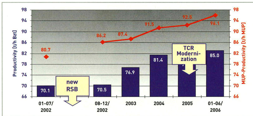
Bild 12: Vorteile des Dreiwälzenverfahrens (Beispiel von Moos Stahl).
