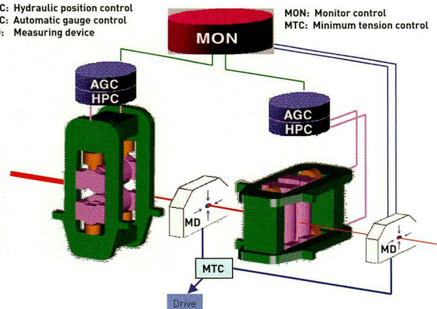
Bild 10: Regeltechnisches Masswalzsystem.
