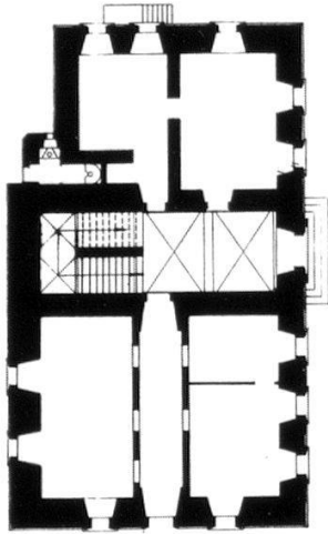
Abb. 58. Grundriß, Erdgeschoß
