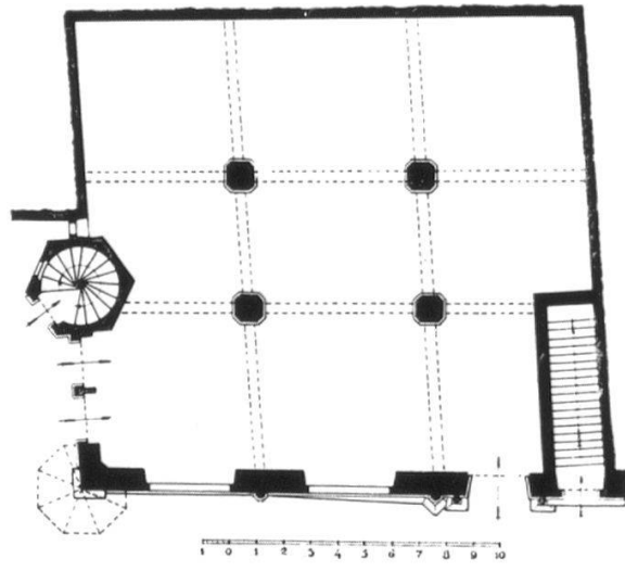
Abb. 29. Grundriß, Erdgeschoß
