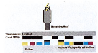
Prinzipschema des Thermo-Druck
