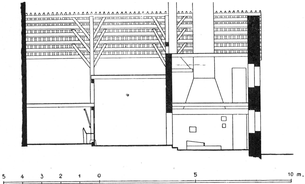
FIG. 8. — Bernex. Coupe.
