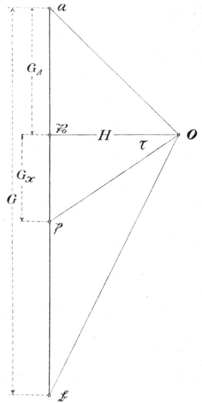
Fig. 1. b Kräftepolygon
