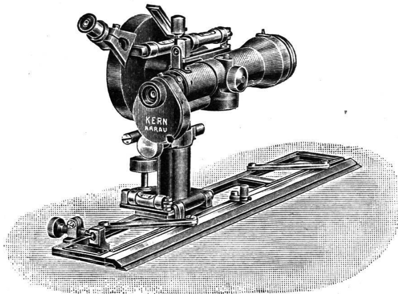
Kippregel Nr. 79
