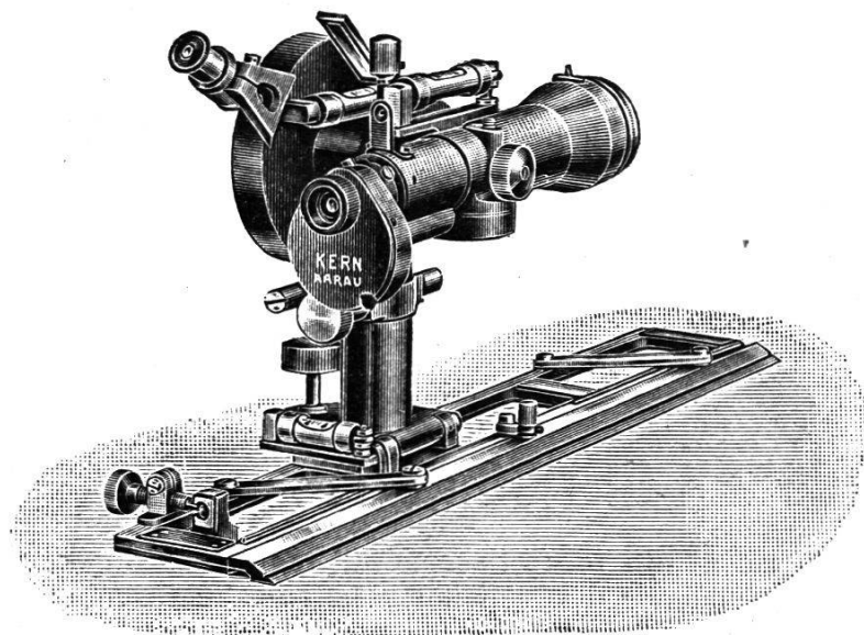
Kippregel Nr. 79
