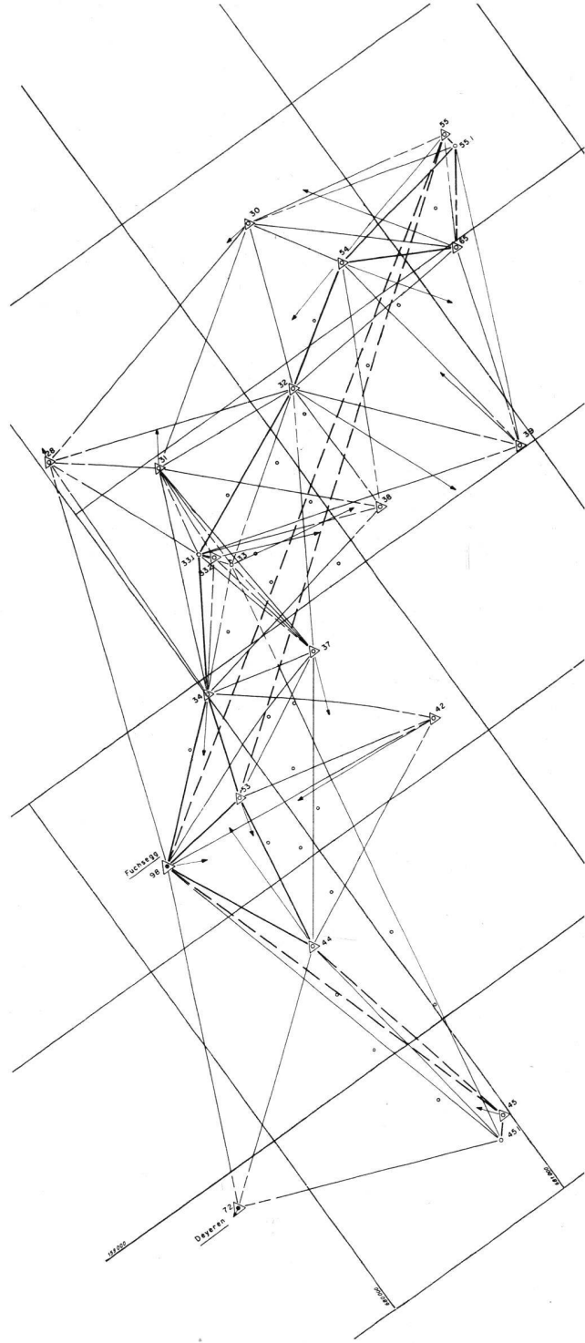
Abb. 6 Restfehlervektoren der Helmerttransformation des freien Netzes auf die Punkte 72, 45, 98, 53, 28, 30, 31, 38, 39
