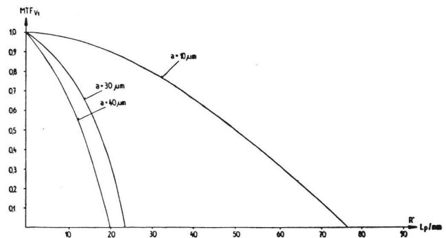
Abb. 13 MTF der durch Vibrationen bedingten Bildverschmierung
