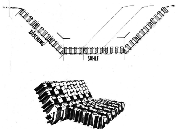
Abb. 1 Normal-Einbauplan
