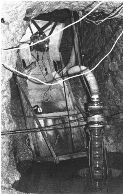
Fig. 1 Le wagonnet du funiculaire et la pompe pour l'évacuation de l'eau au bas de la galerie inclinée.
