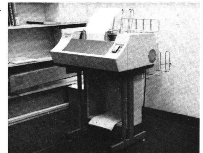
Trommelplotter Calcomp 936 mit 3 Federn für Papier oder Folie von 86 cm Breite, auf 0,05 mm positionierbar, Geschwindigkeit 10 cm/Sek unabhängig von der Liniengeometrie
