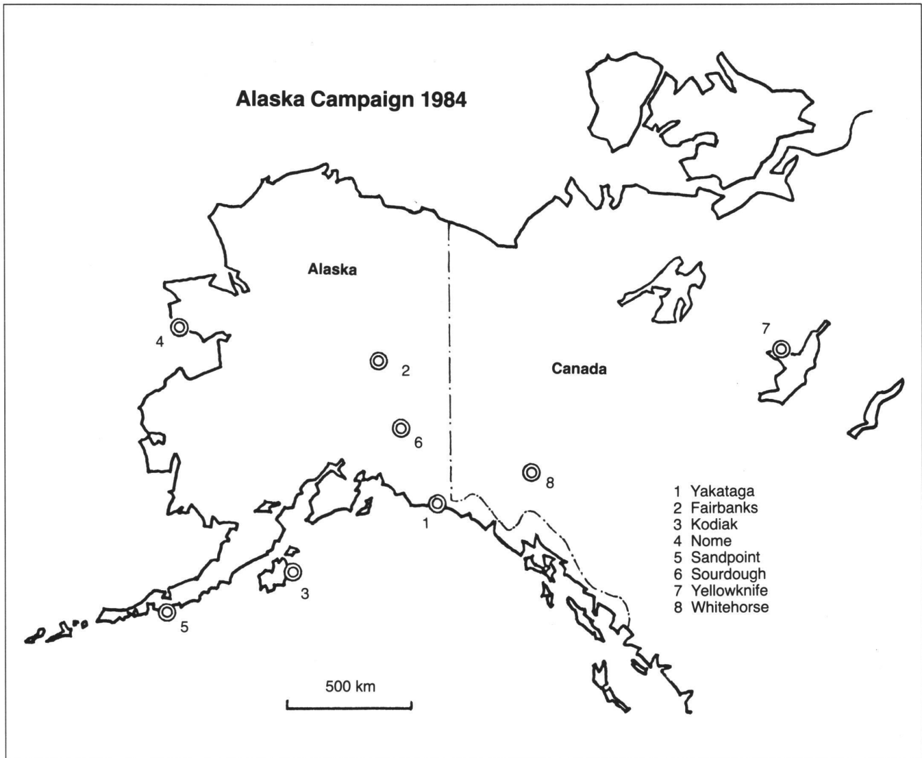
Abb. 1: The 1984-Alaska-GPS-Campaign
