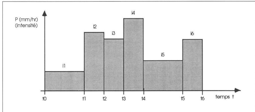
Fig. 5: Discretisation de la pluie observée
