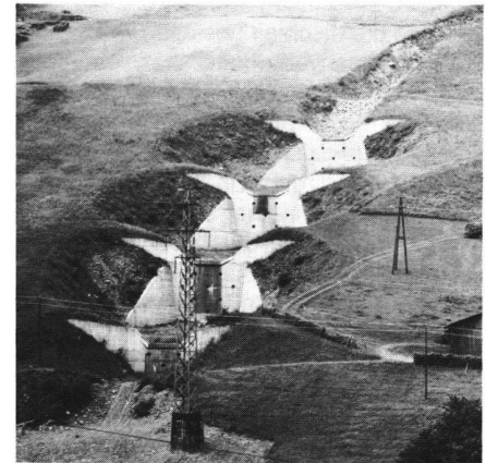
Abb. 6: Die drei Murablagebecken mit Absturzsperren im Wassertobel der Gemeinde Tschagguns.
