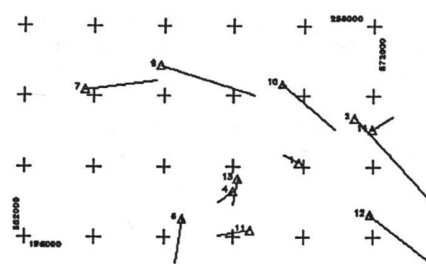
Abb. 5: Lagedifferenzen zwischen Karte und Orthophoto. Massstab der Vektoren: |—| = 6 m.
