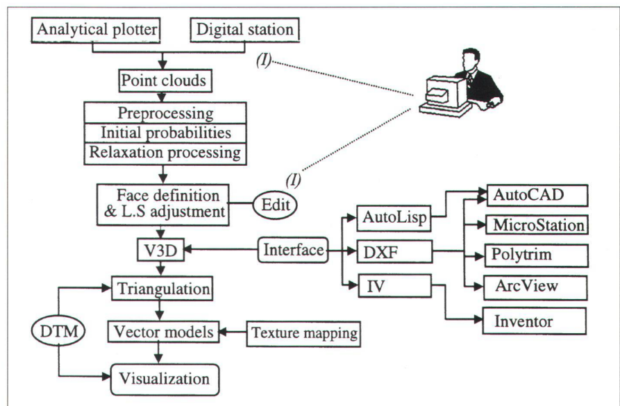
Abb. 2: Komponenten des CyberCity Modelers.
