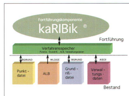
Abb. 3: Datenfluss zwischen Fortführung und Datenhaltung.
