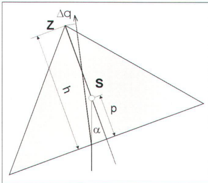
Abb. 2: Querabweichung bei verschwenktem Prisma (Prinzipskizze).
