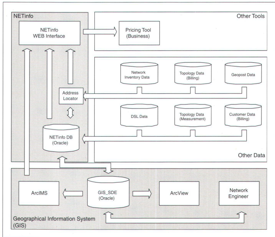
Abb. 5: NETinfo: Systemarchitektur.
