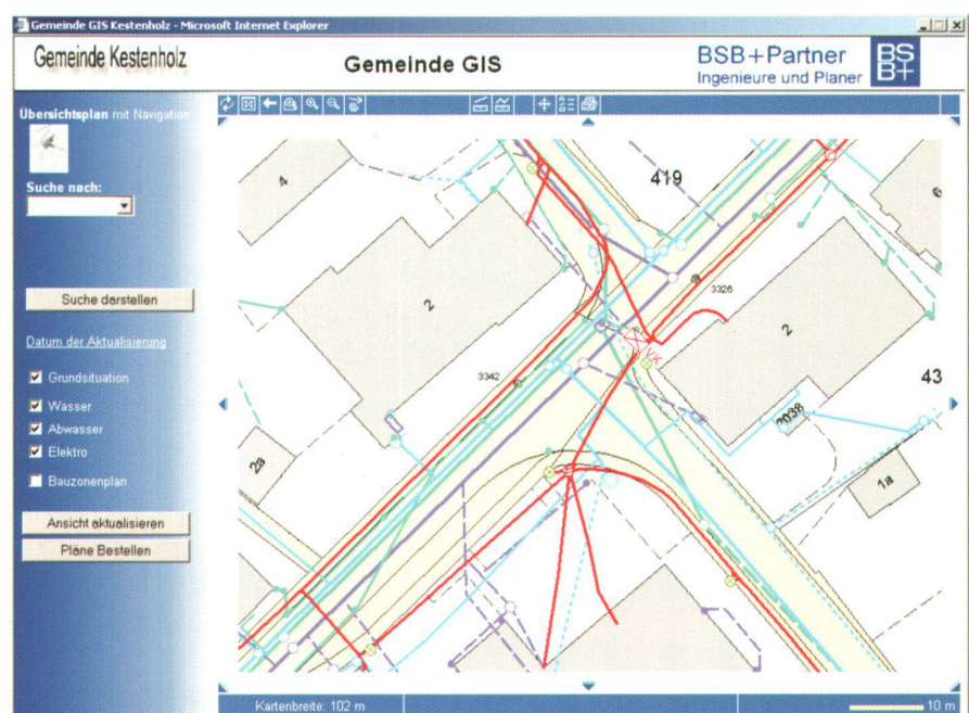
Abb. 7: Web-GIS Kestenholz: Ausschnitt aus Leitungskatasterplan.
