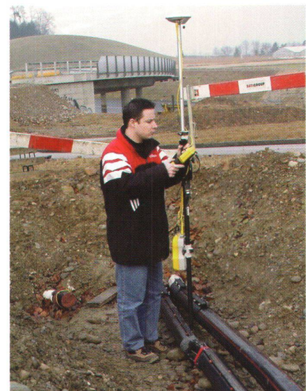
Abb. 10: Positionierung mit swipos-GIS/GEO.
