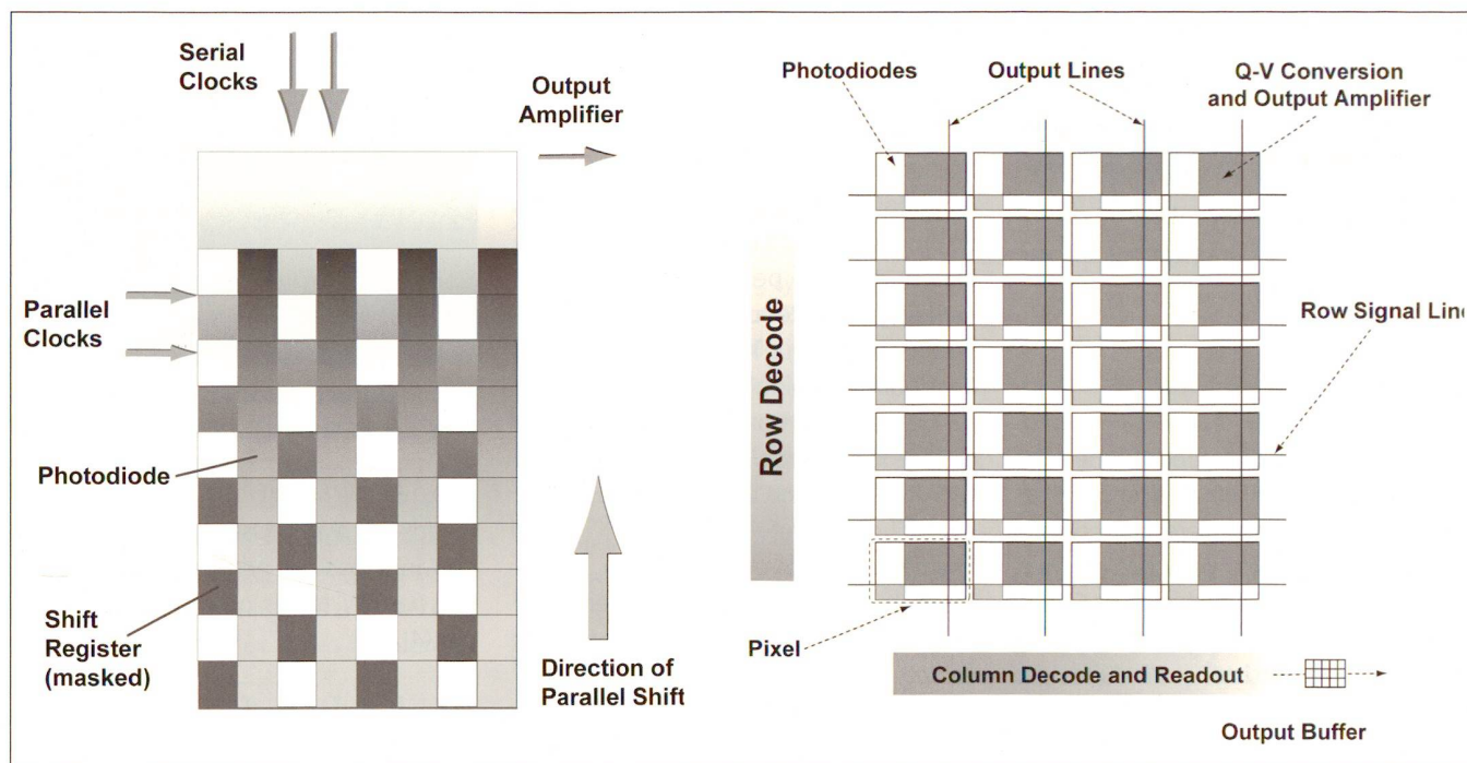
Fig. 2: Architecture CCD (gauche) et CMOS (droite).
