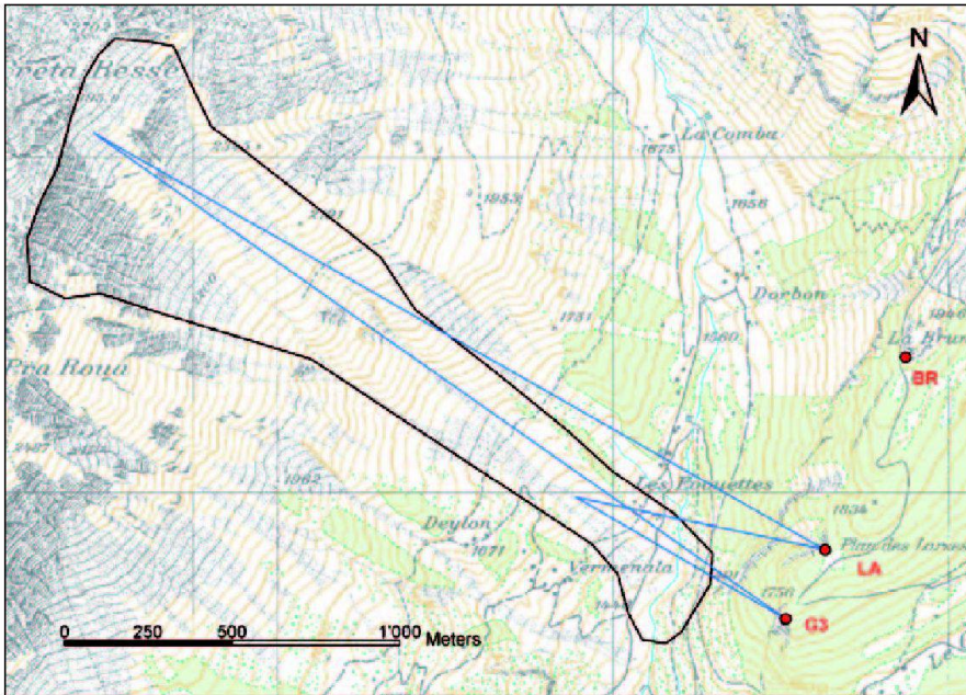
Abb. 1: Die möglichen Kamera-Standpunkte G3, LA und BR (rot) mit den Visuren ins Anriss- und Ablagerungsgebiet (blau) und dem Gefahrenbereich der Lawine (schwarz). Reproduziert mit Bewilligung von swisstopo (BA071266).
