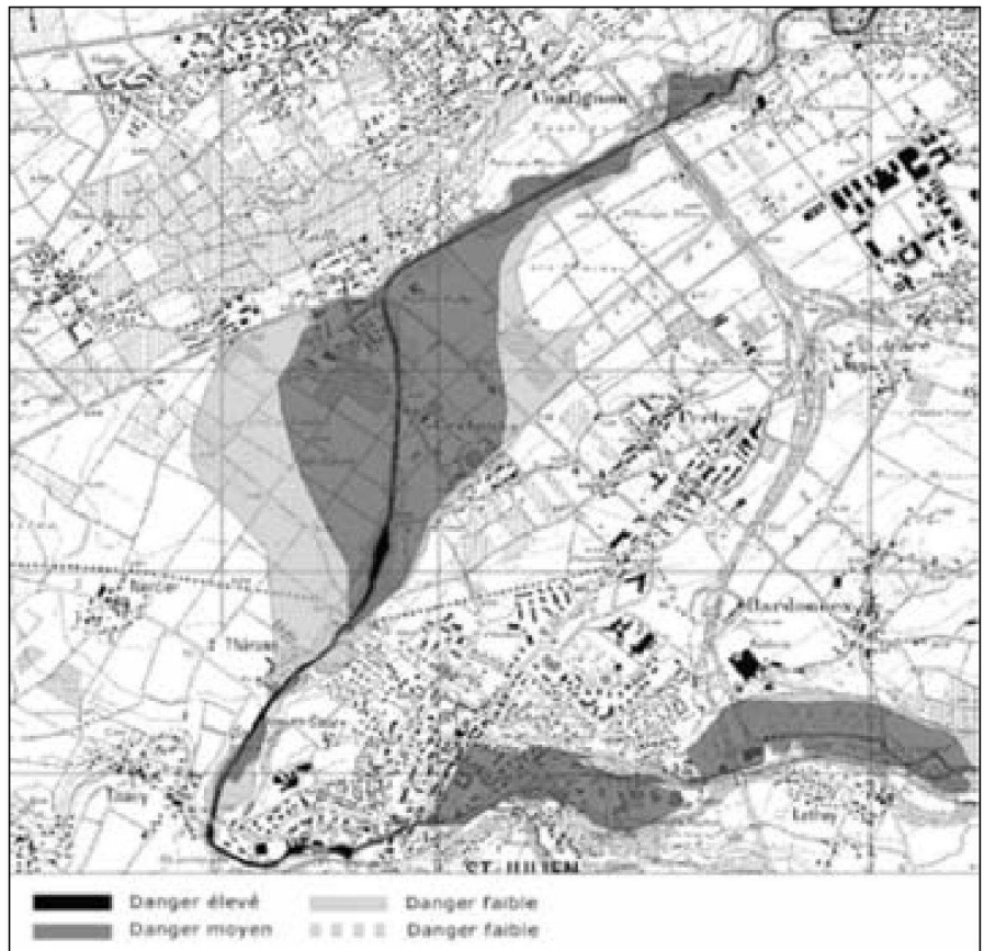
Fig. 2: Carte de dangers de Lully, région de Genève, parue 2000.
