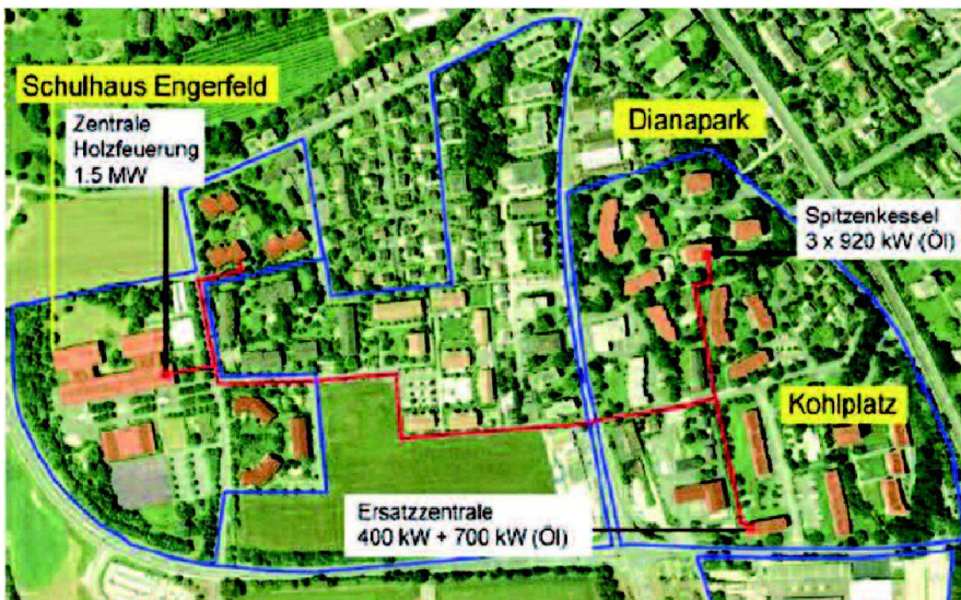
Abb. 2: Wärmeverbund Engerfeld.
