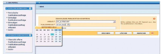
Abb. 2: Web-Applikation «Geodaten-Publikation».
